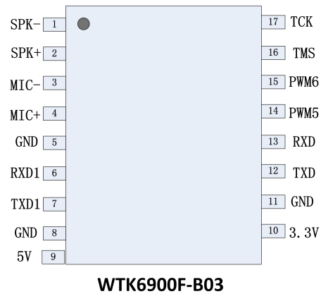
图表 3 - WTK6900F-B03 模块管脚分布
