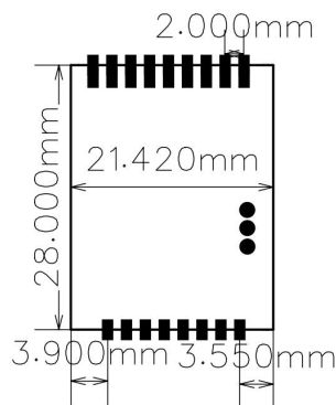
图表 2 - WTK6900F-B03 模块尺寸图
