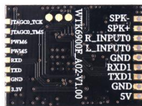
背面
